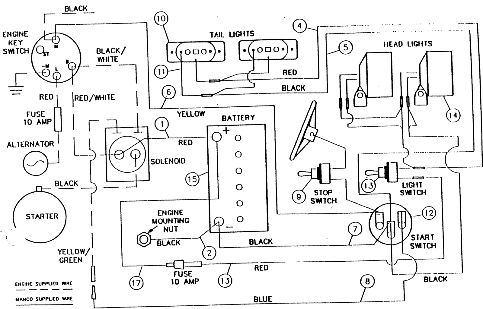
609 WIRING DIAGRAM
